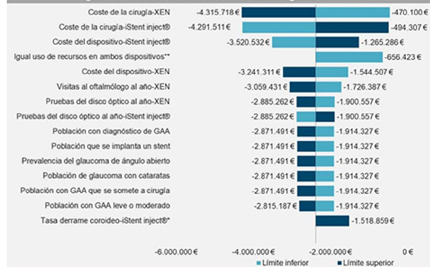
Figura 4. Análisis de sensibilidad univariado. Diagrama de tornado
